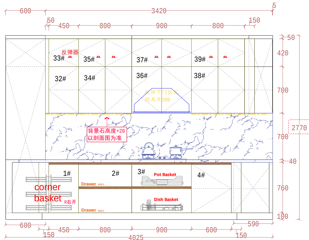
ELEVATION B
