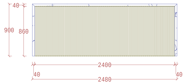
ELEVATION G
