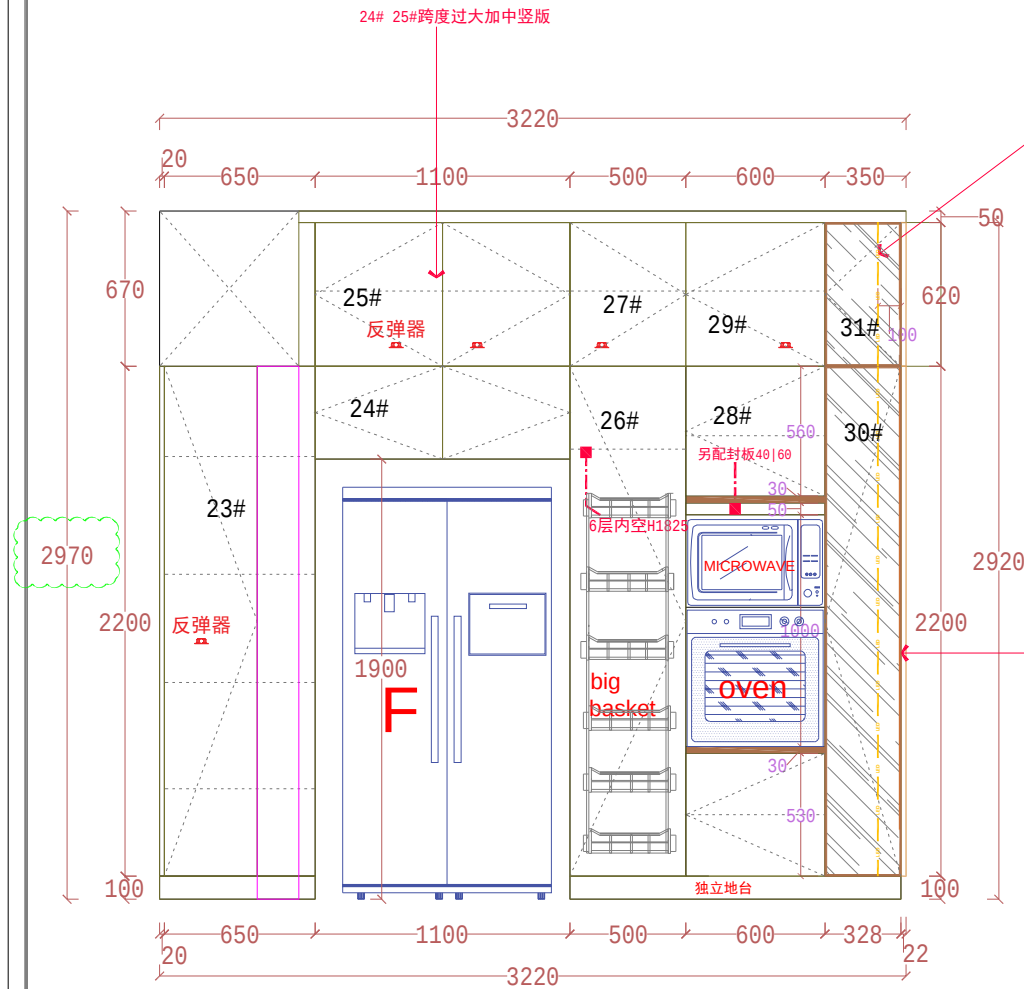
ELEVATION E
