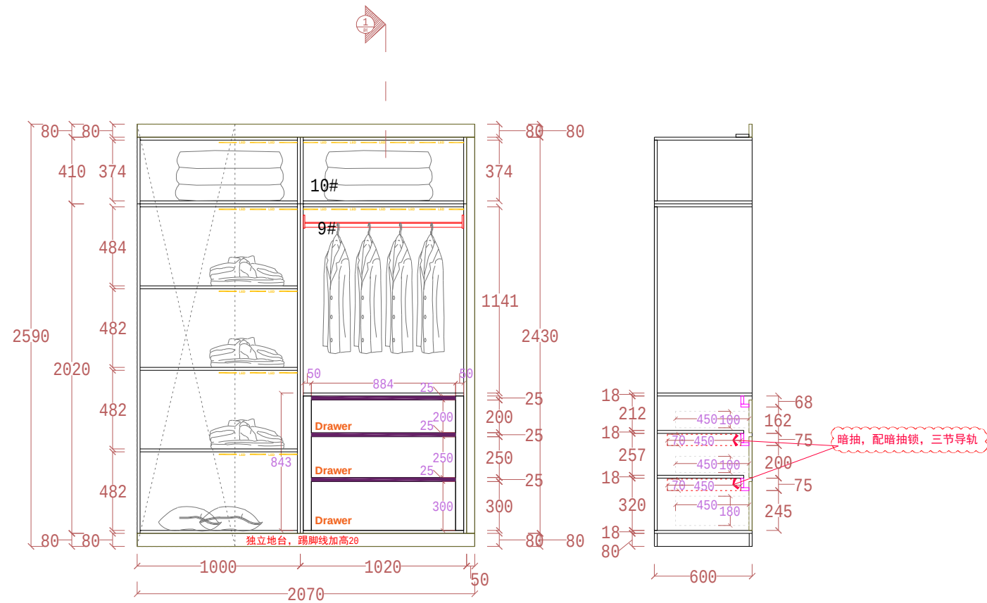
ELEVATION B
